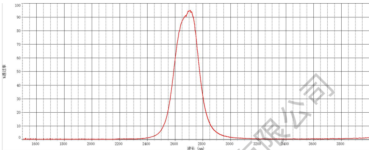
2.70um 红外窄带滤光片透射曲线图
