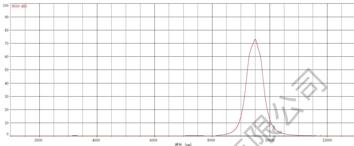
9. 50um 红外窄带滤光片透射曲线图
